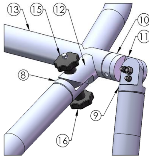
Узел Верхней Секции
