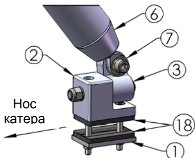
Узел Основания (Задний)
