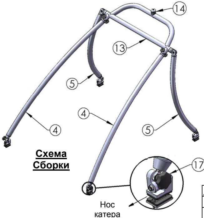
Узел Основания (Передний)
